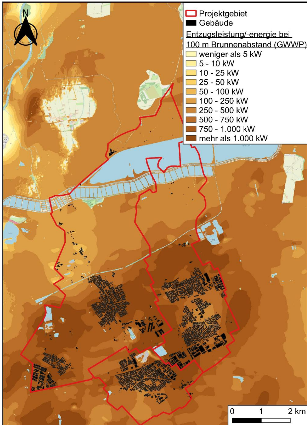
Abbildung 38: Entzugsleistungen bei 100 m Brunnenabstand Quelle: Bayerisches Landesamt für Umwelt
