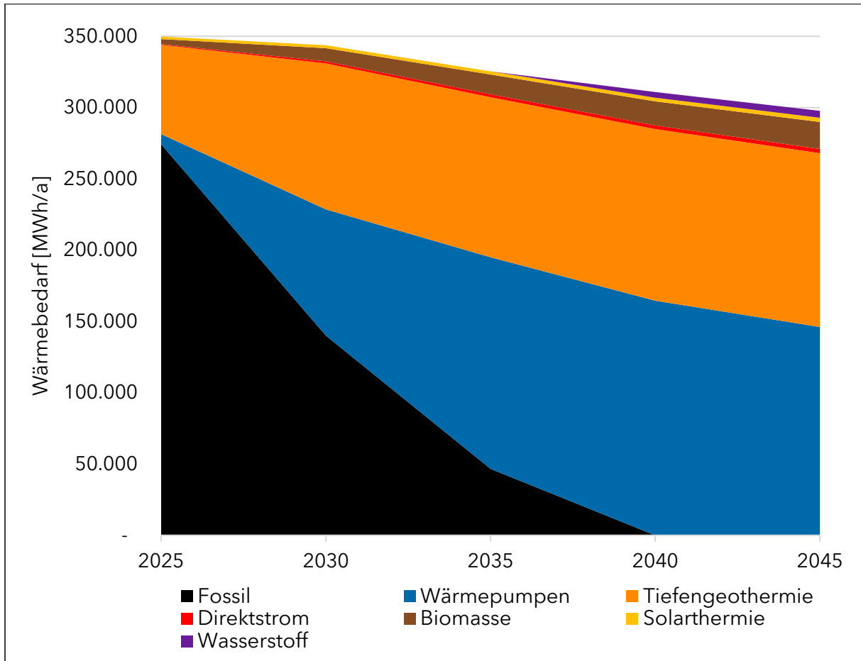
Abbildung 67: Hochlauf der Energieträgerverteilung nach Zielszenario bis 2045
