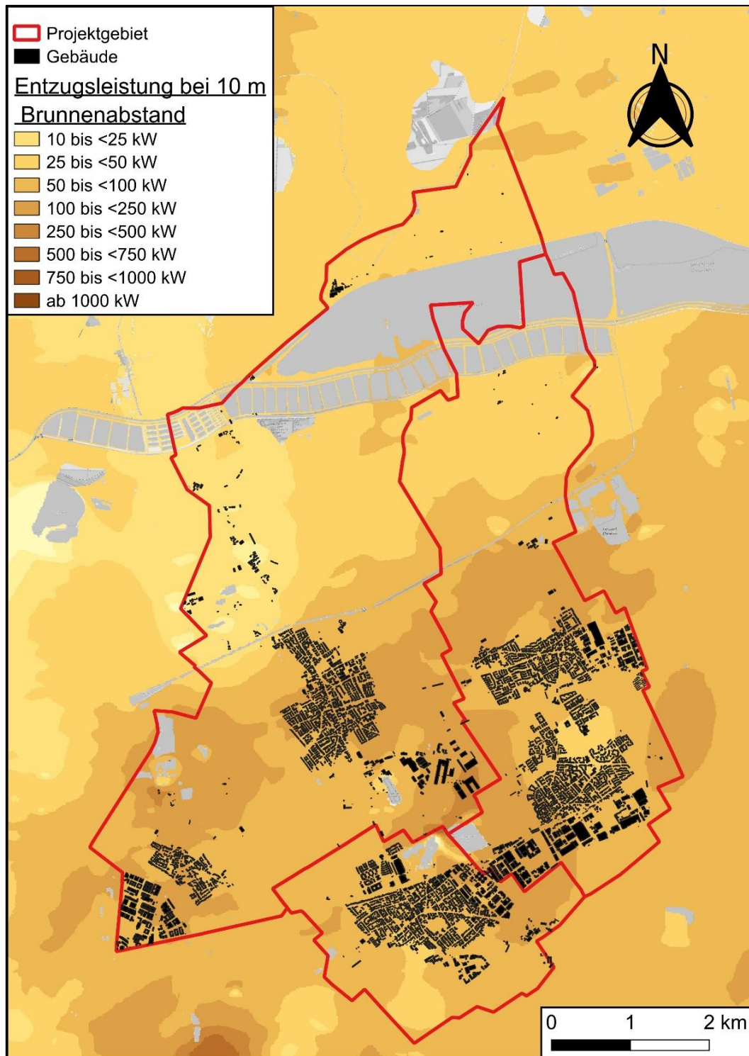
Abbildung 39: Entzugsleistungen bei 10 m Brunnenabstand Quelle: Bayerisches Landesamt für Umwelt
