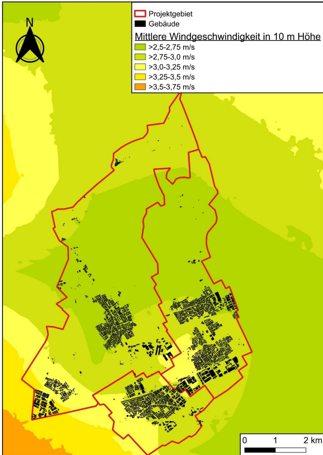
Abbildung 54: Mittlere Windgeschwindigkeiten in 10 m Höhe Datenquelle: energieatlas.bayern.de
