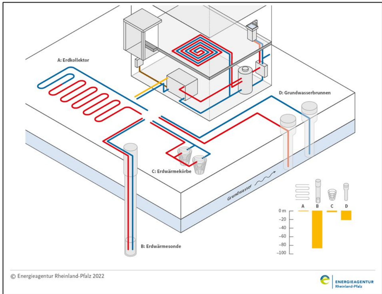
Abbildung 31: Überblick über Wärmeentzugstechnologien zur Nutzung oberflächennaher Geothermie
