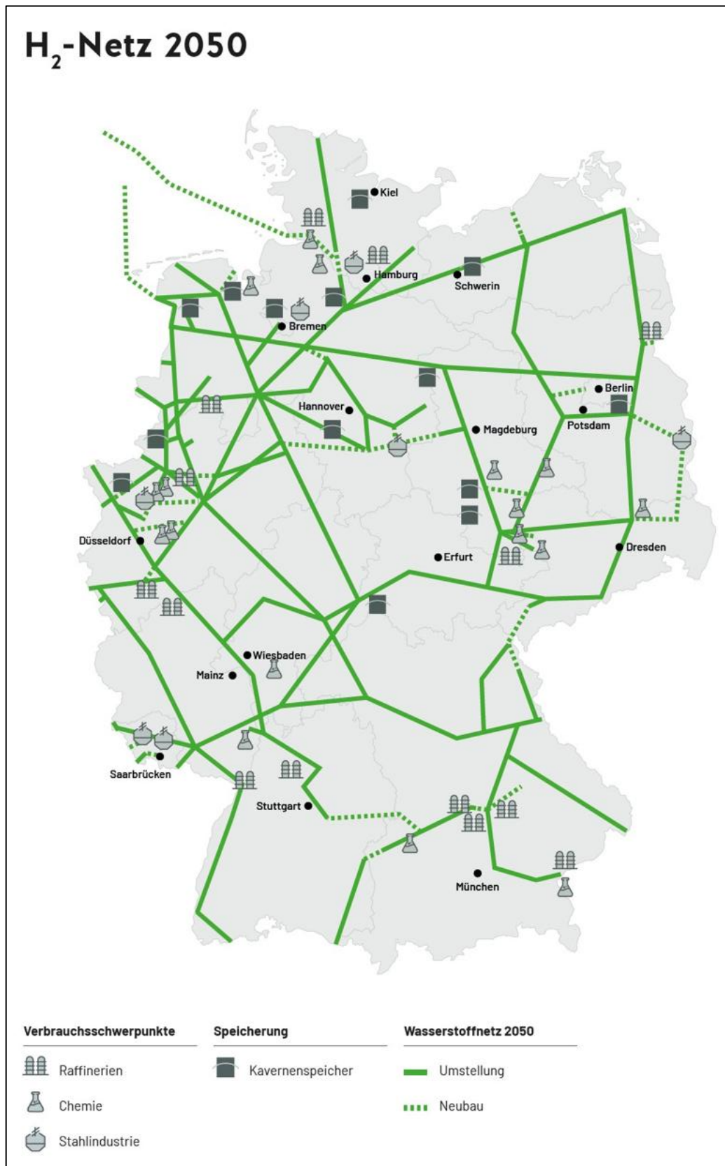
Abbildung 52: Geplantes Wasserstoffnetz 2050 Quelle: fnb-gas.de
