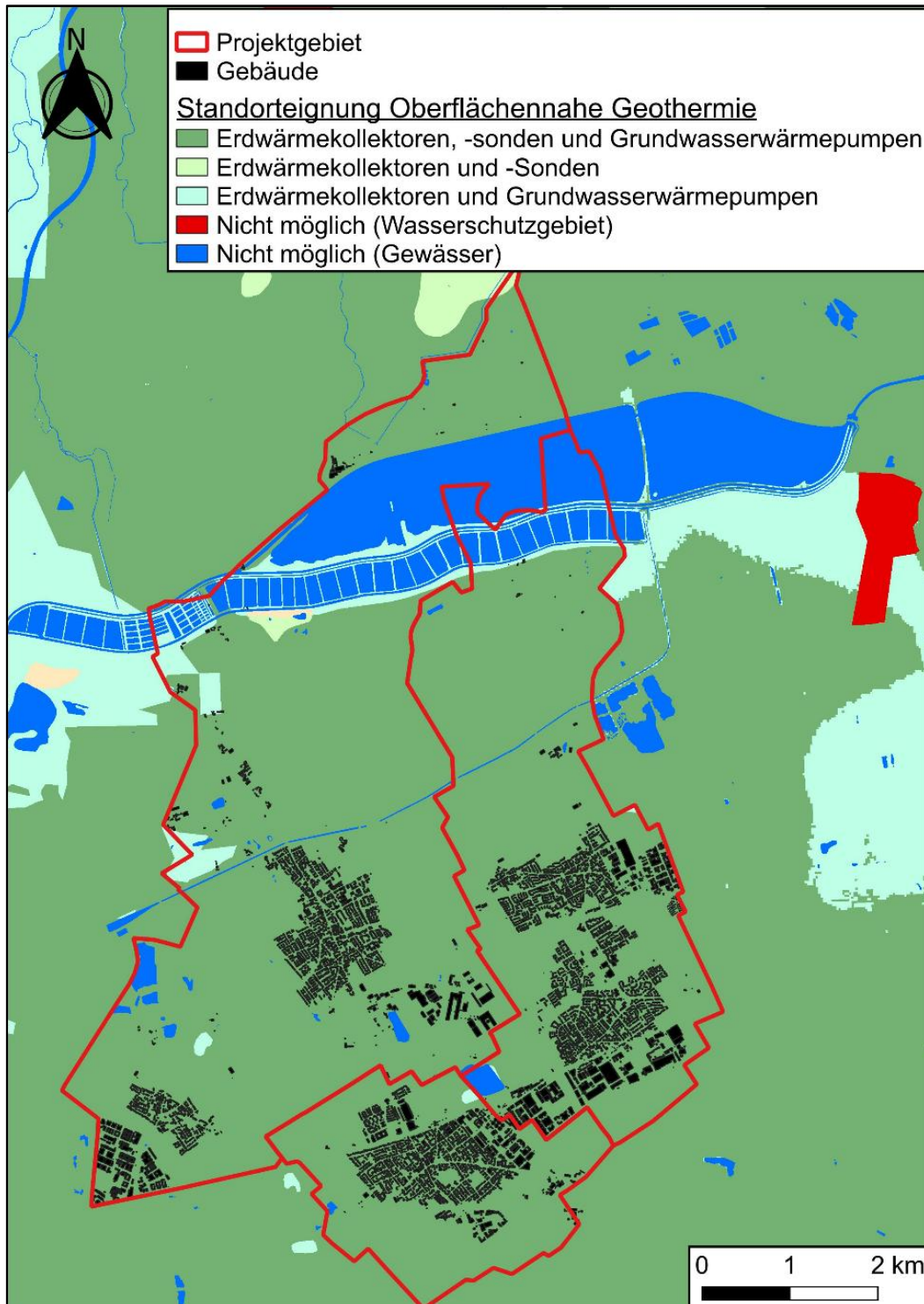
Abbildung 33: Standorteignung für oberflächennahe Geothermie Quelle: Bayerisches Landesamt für Umwelt
