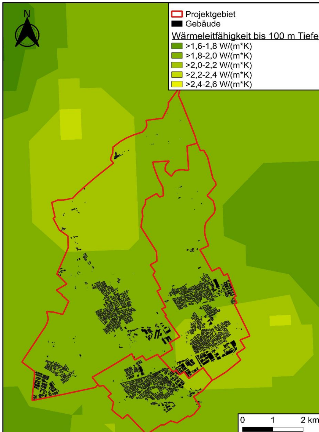
Abbildung 34: Wärmeleitfähigkeit im Projektgebiet bis 100 m Tiefe Quelle: Bayerisches Landesamt für Umwelt
