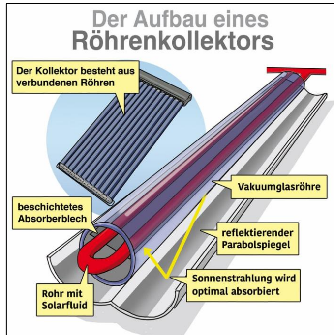
Abbildung 28: Aufbau eines Röhrenkollektors Quelle: solaranlage-ratgeber.de
