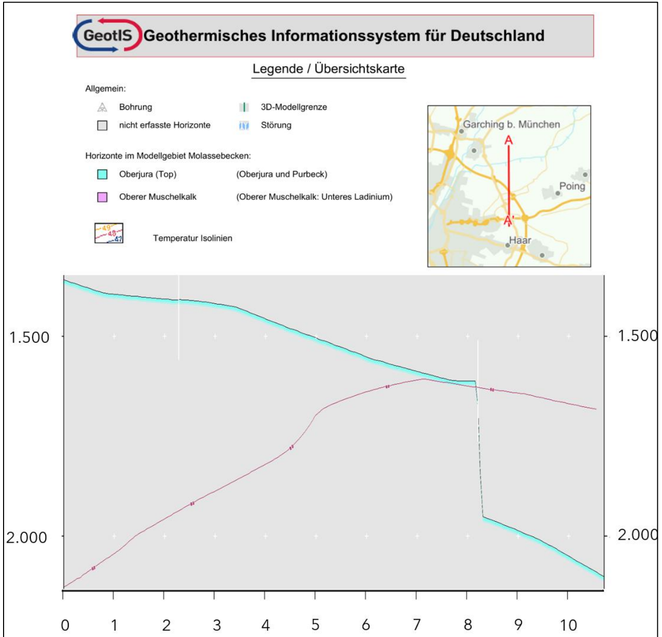
Abbildung 48: Tiefenlokalisierung des vorhandenen Aquifers für tiefengeothermische Energienutzung. Quelle: GeotIS
