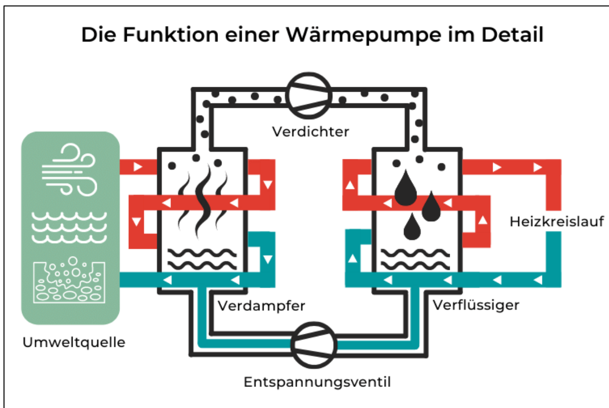
Abbildung 32: Funktionsprinzip einer Wärmepumpe Quelle: solarwatt.de
