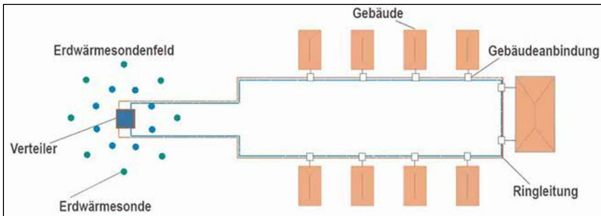
Abbildung 42: Beispiel für ein kaltes Nahwärmenetz. Quelle: Energieagentur Rheinland-Pfalz GmbH
