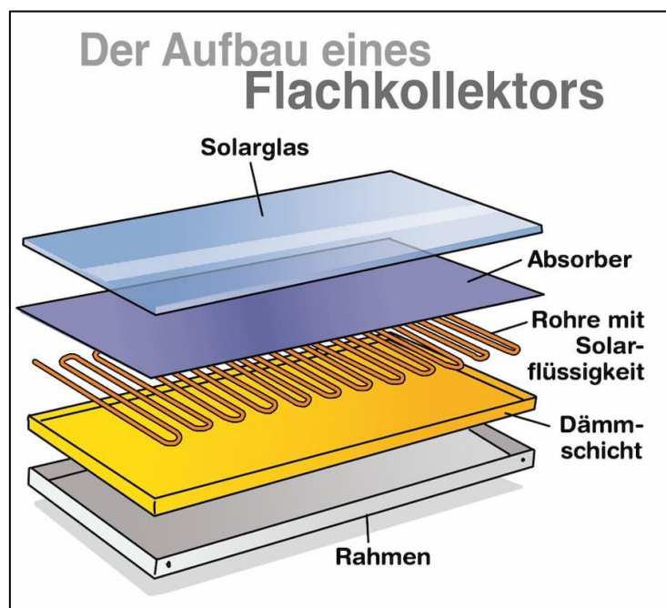
Abbildung 27: Aufbau eines Flachkollektors Quelle: solaranlage-ratgeber.de
