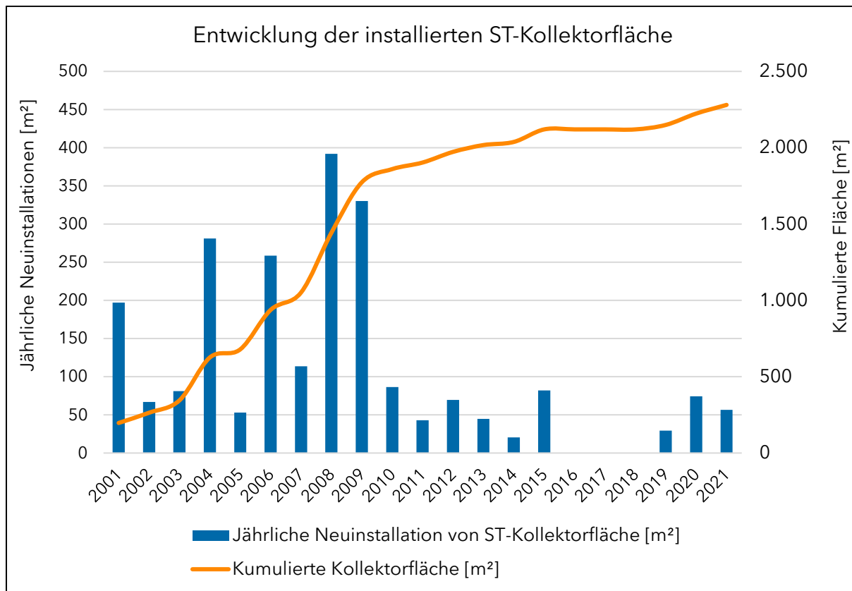
Abbildung 11: Hochlauf der installierten Kollektorfläche von Solarthermie seit 2001 Quelle: Solaratlas.de
