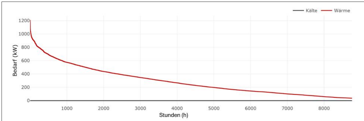
Abbildung 62: Ermittelte Jahresdauerlinie des Gewerbegebietes bei einer simulierten Anschlussquote von 70 %
