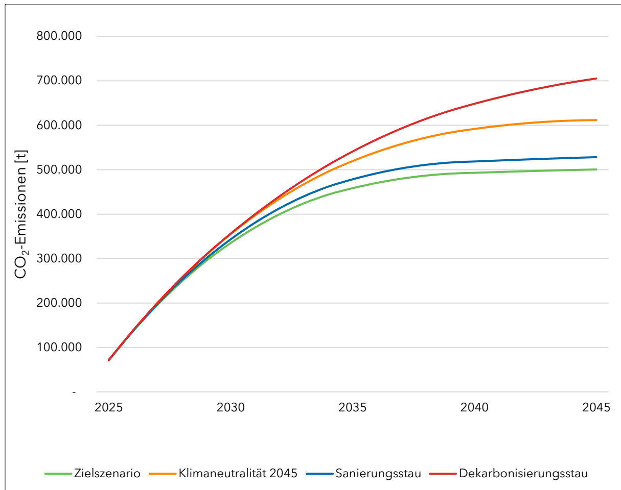
Abbildung 70: Kumulierte CO 2 -Emissionen für die einzelnen Szenarien
