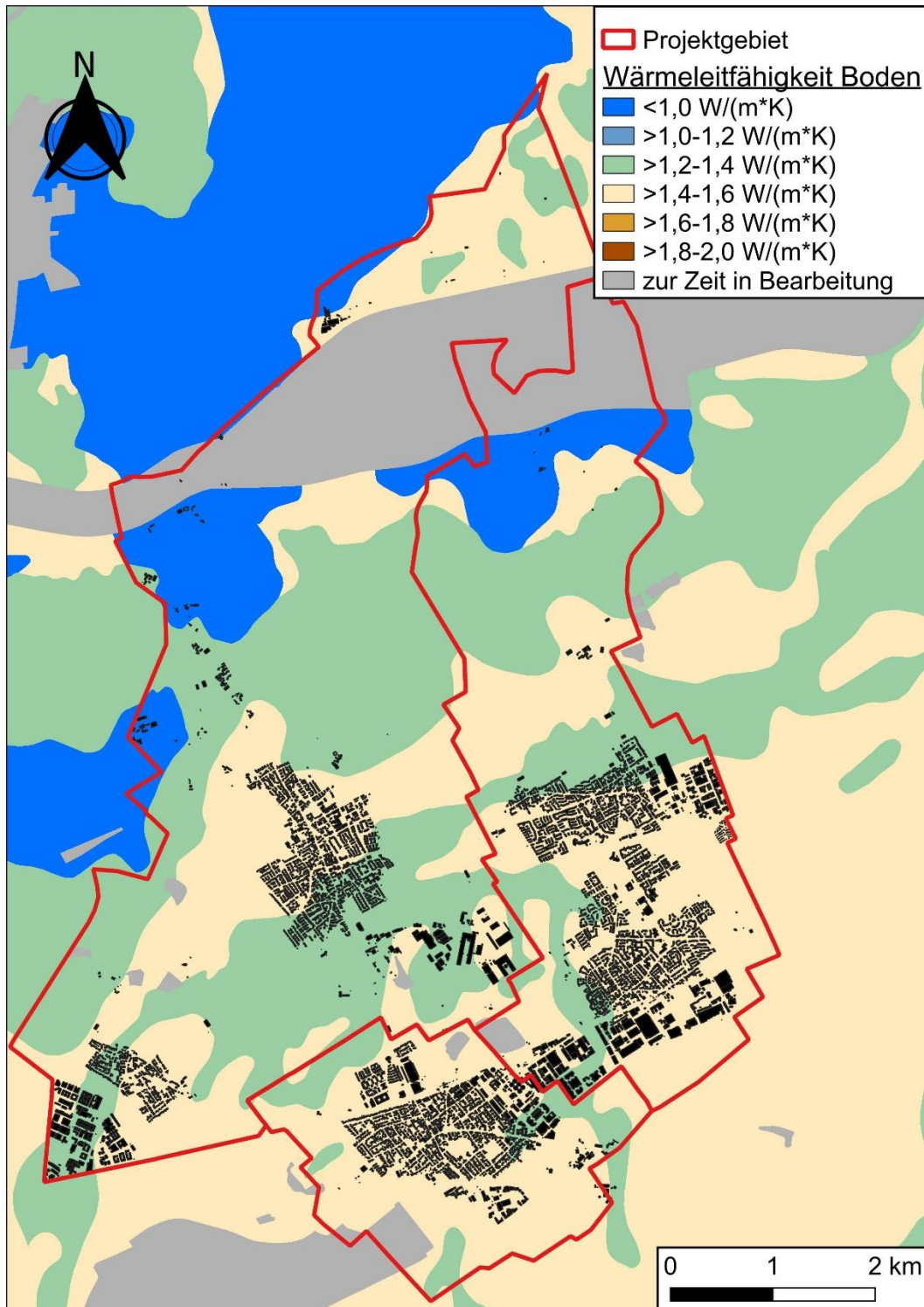
Abbildung 35: Spezifische Wärmeleitfähigkeit bis 2 m Tiefe Quelle: Bayerisches Landesamt für Umwelt
