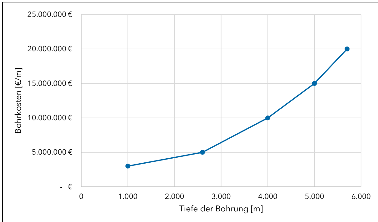
Abbildung 50: Kostenfunktion der Bohrkosten für eine Tiefengeothermieanlage. Datenquelle: AGFW Praxisleitfaden Tiefengeothermie
