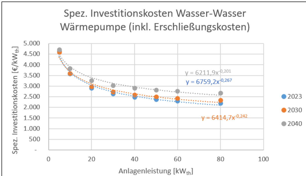
Abbildung 40: Investitionskosten für Grundwasserwärmepumpen gemäß Prognos AG et al.
