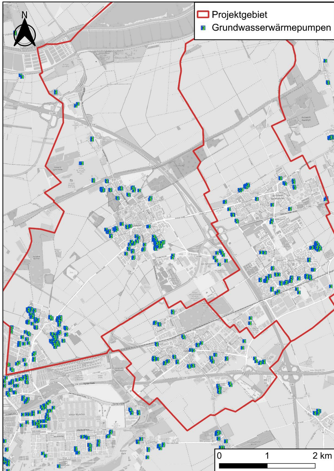
Abbildung 13: Erdwärmesonden und Grundwasserwärmepumpen Datenquelle: Energieatlas Bayern
