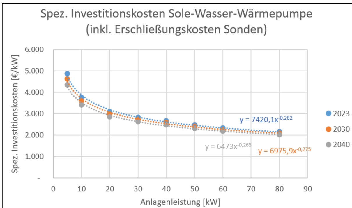
Abbildung 41: Investitionskosten für Sole-Wasser Wärmepumpen (Erdsonden) gemäß Prognos AG et al.
