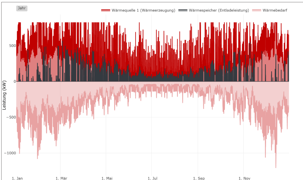
Abbildung 63: Abdeckung des Lastprofils des Gewerbegebietes in Feldkirchen durch die Grundwasserwärmepumpe und einem Pufferspeicher
