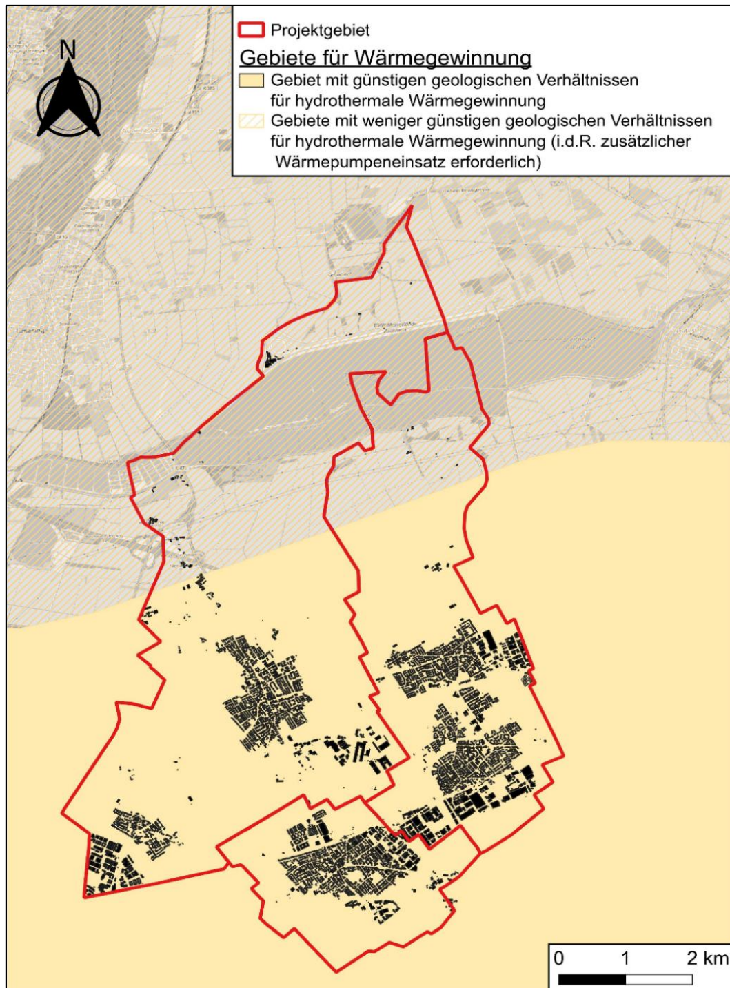
Abbildung 47: Übersicht der möglichen Gebiete für Tiefengeothermie im Projektgebiet. Datenquelle: Energie-Atlas Bayern, Kartenhintergrund: OpenStreetMaps
