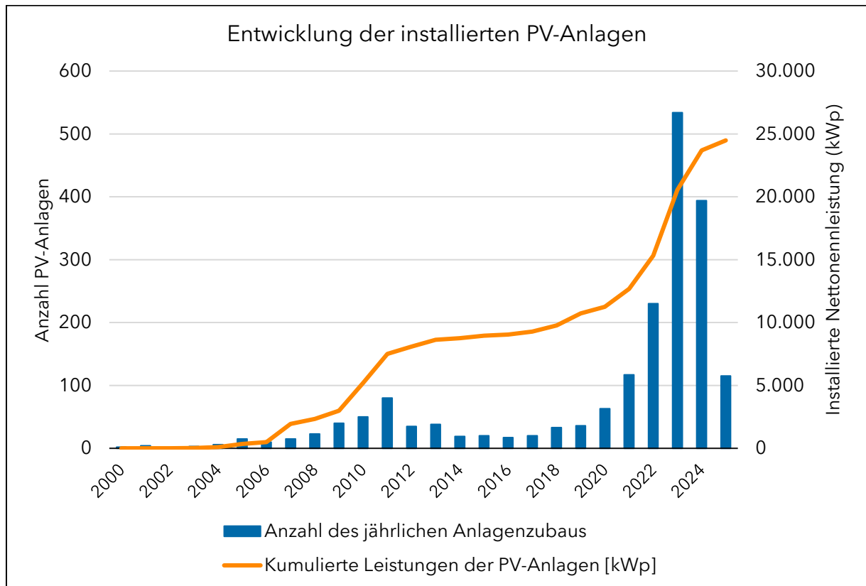
Abbildung 12: Hochlauf der installierten PV-Anlagen und der kumulierten Leistung seit 2000 Quelle: Marktstammdatenregister
