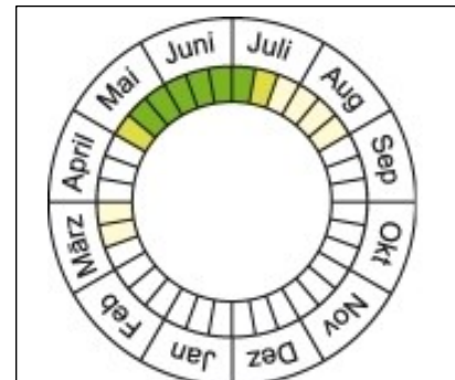
Abb. 4: Brutzeit-Diagramm Feldlerche gemäß BAYLfU (2023).
