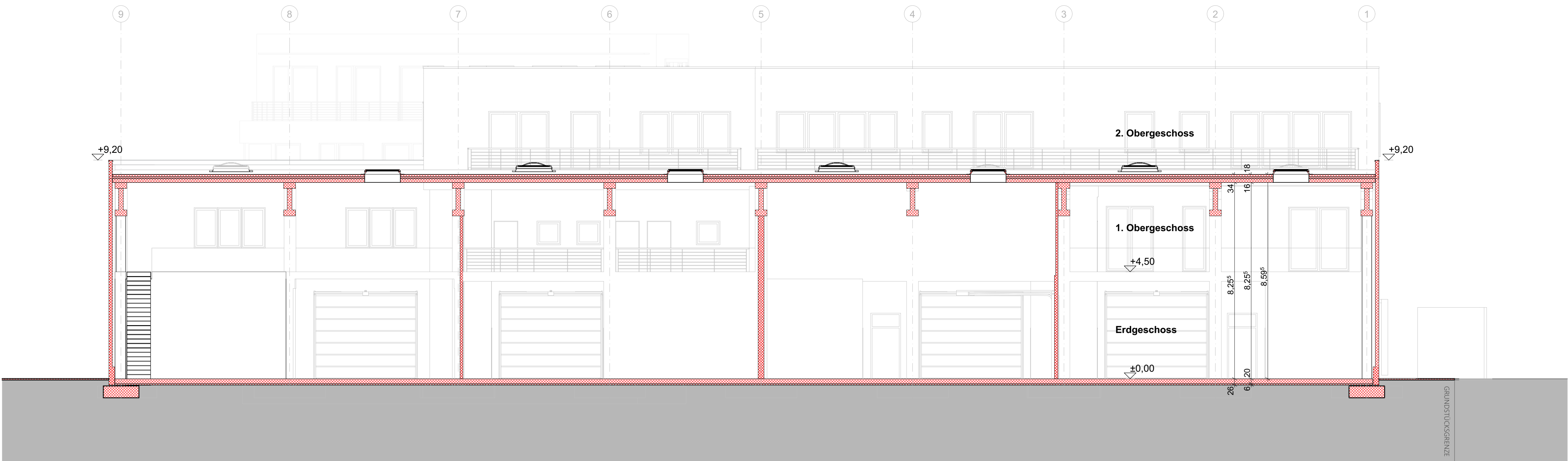
Schnitt 8
