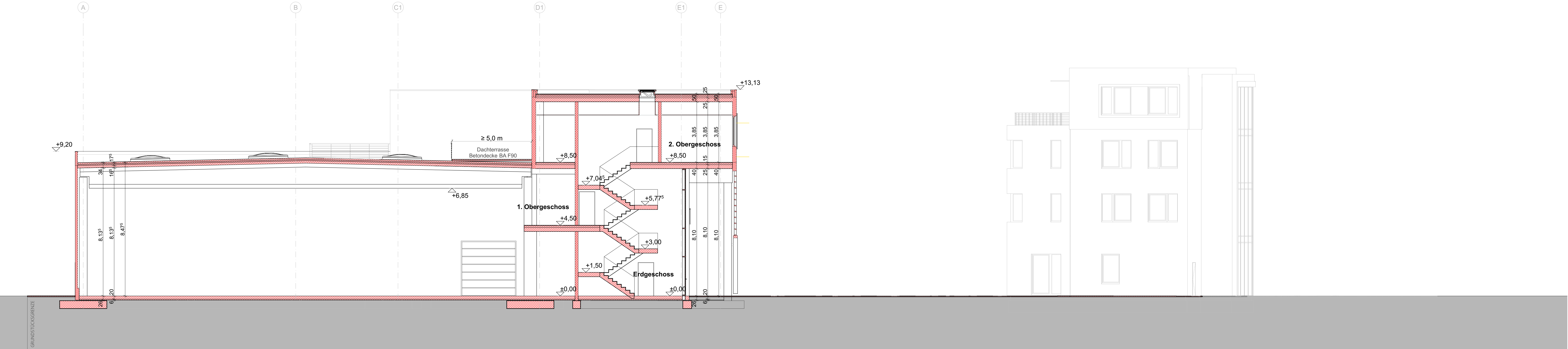
Schnitt 5
