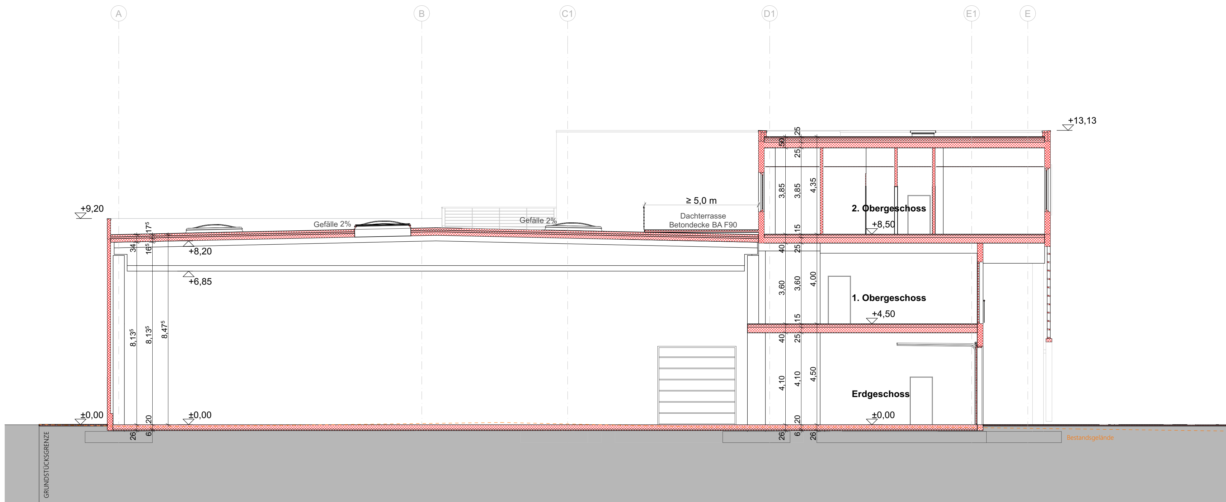
Schnitt 4
