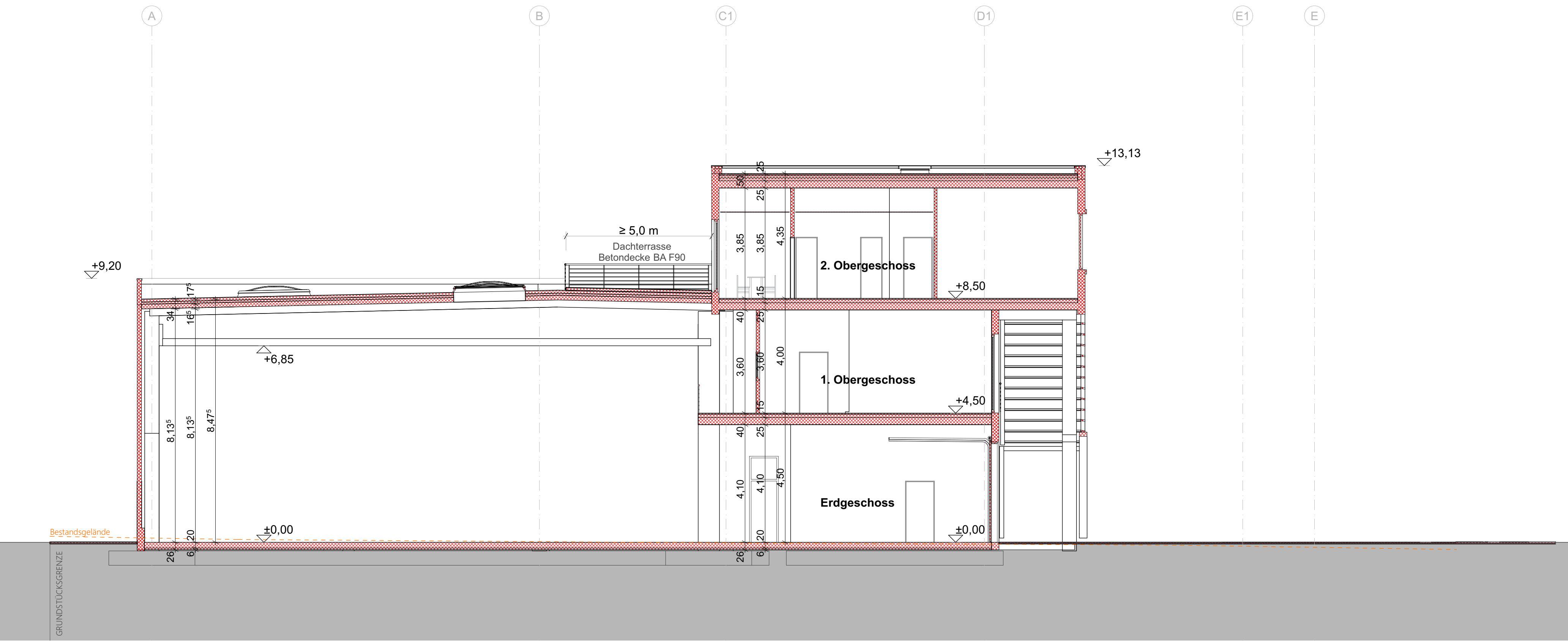
Schnitt 6
