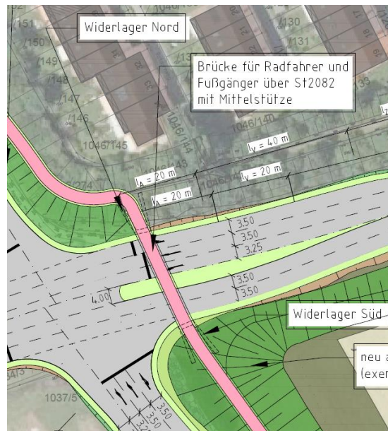
Abbildung 3 Höhenfreie Querung
